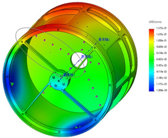
(b) 位移分布 (b) Displacement distribution
