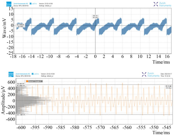
图 16 乙烷吸收信号和谐波信号 Fig. 16 Ethane absorption signal and harmonic signal
