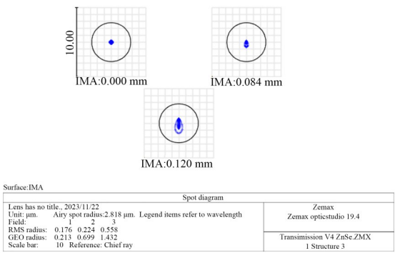
图 9 发射系统点列图
