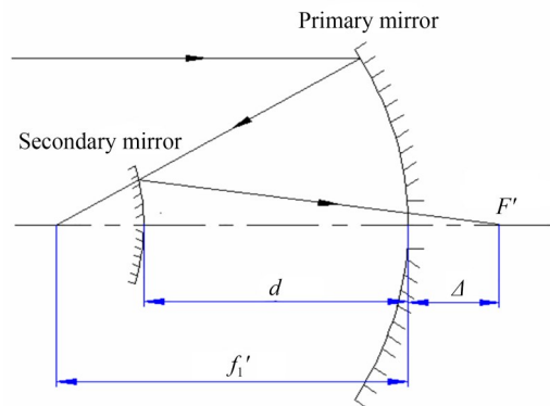
图6 经典的卡塞格林系统示意图
