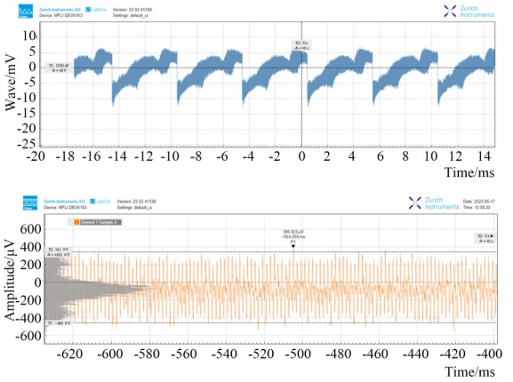
图 15 甲烷吸收信号和谐波信号 Fig. 15 Methane absorption signal and harmonic signal
