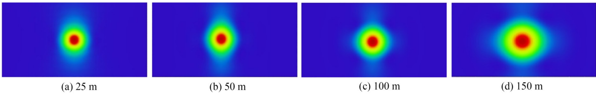
图 10 不同位置的发射光斑示意图 Fig. 10 Schematic diagram of emission spot at different positions
