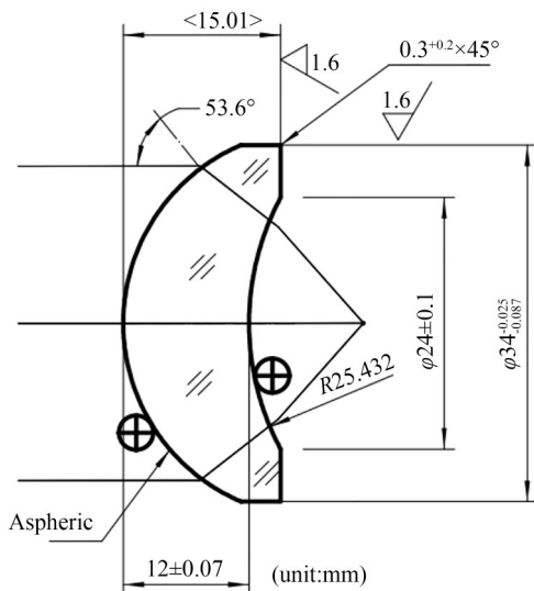
图5 发射镜设计
