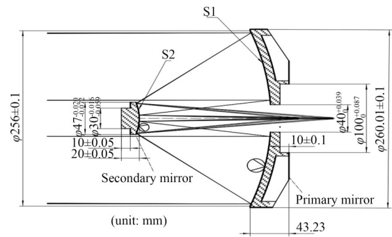
图 7 接收光路
