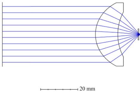
图 8 激光准直系统结构
